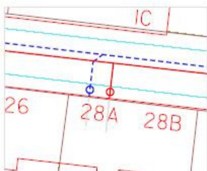
Tilslutningsprincip med spildevand og regnvandsskelbrønd hvor bebyggelse er i skel
